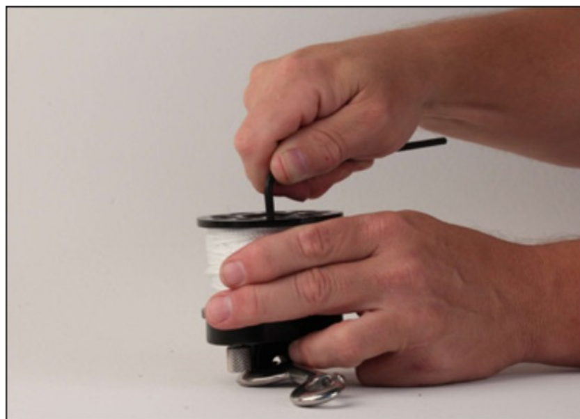
Instalacja/deinstalacja adaptera EasyGrip™
